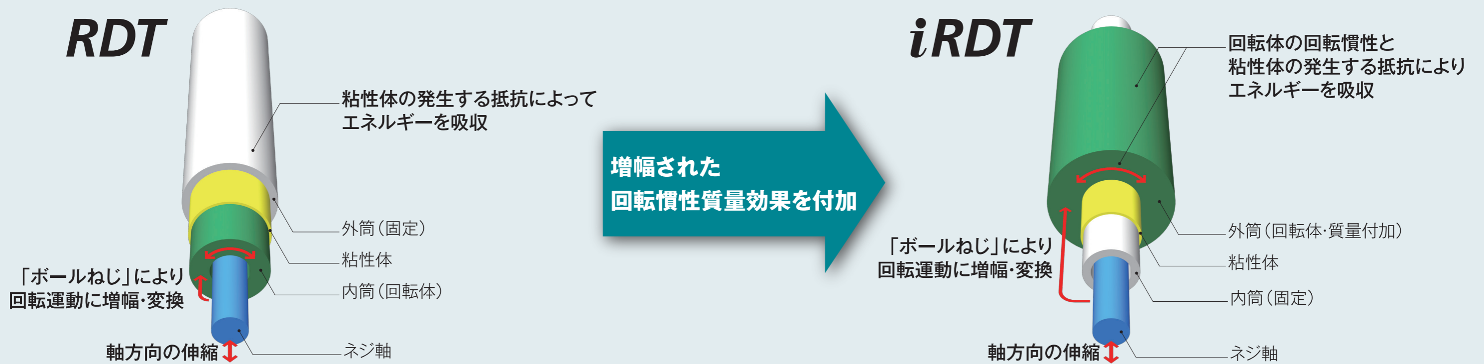
減衰こま(RDT)と慣性こま(iRDT)の基本構造と作動原理
